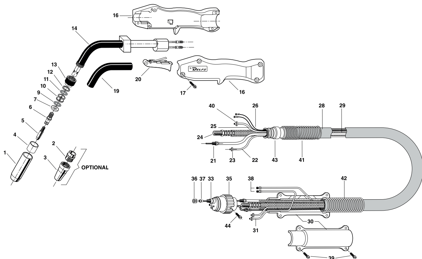
LISTA RICAMBI
